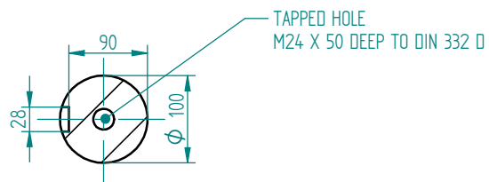
Przekrój A-A 1:5
